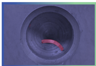
切粉検査
