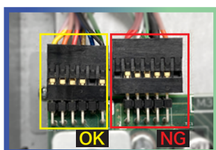
挿入検査
