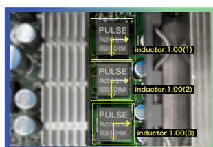
組立検査
